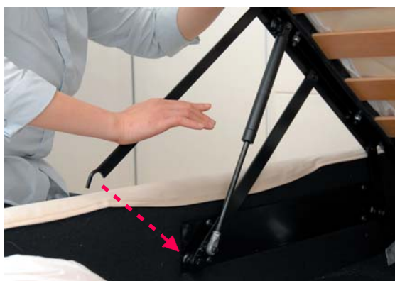
在氣壓支撐旁額外添加活動金屬支撐，擺放物品時可更放心。
